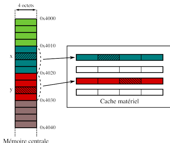
FIGURE 2.1 – Effets sur le cache de la lecture de x et y
